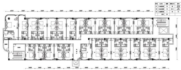
酒店四层平面布置图
